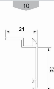
روکوب ۳۰ Suppressed the binding Code : 10022 weight : 0.22 kg/m
