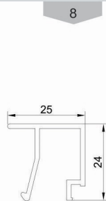
زهوار ۲ جداره ترمال Double rickety Code : 21352 weight : 0.31 kg/m
