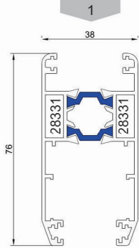
پروفیل لنگه Vent profile Code : 28331-28331 weight : 1.51 kg/m
