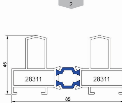
پروفیل فریم Frame profile Code : 28311-28311 weight : 1.65 kg/m
