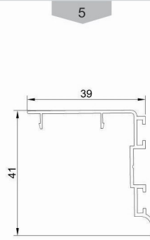
درپوش gap Code : 28321 weight : 0.27 kg/m
