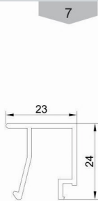
زهوار ۲ جداره ترمال Double rickety Code : 21351 weight : 0.3 kg/m
