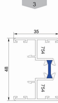
واسطه ۴ لنگه The Middle of four Vent Code : 754-754 weight : 0.75 kg/m
