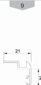
روکوب ۱۴ Suppressed the binding Code : 10021 weight : 0.2 kg/m
