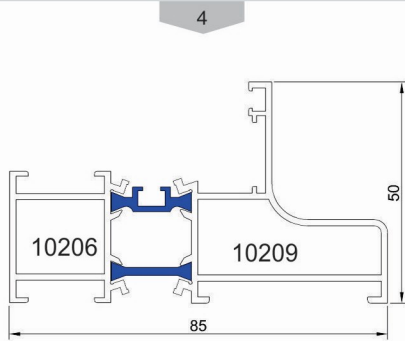
پروفیل فریم Frame profile Code : 10206-10209 weight : 1.42 kg/m
