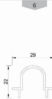
پروفیل وسط ۲ فریم The middle of two Frame Code : 753 weight : 0.24 kg/m
